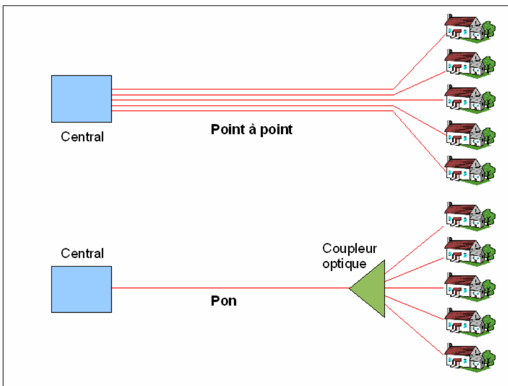
Les deux modes de diffusion : point à point ou point à multipoint.
